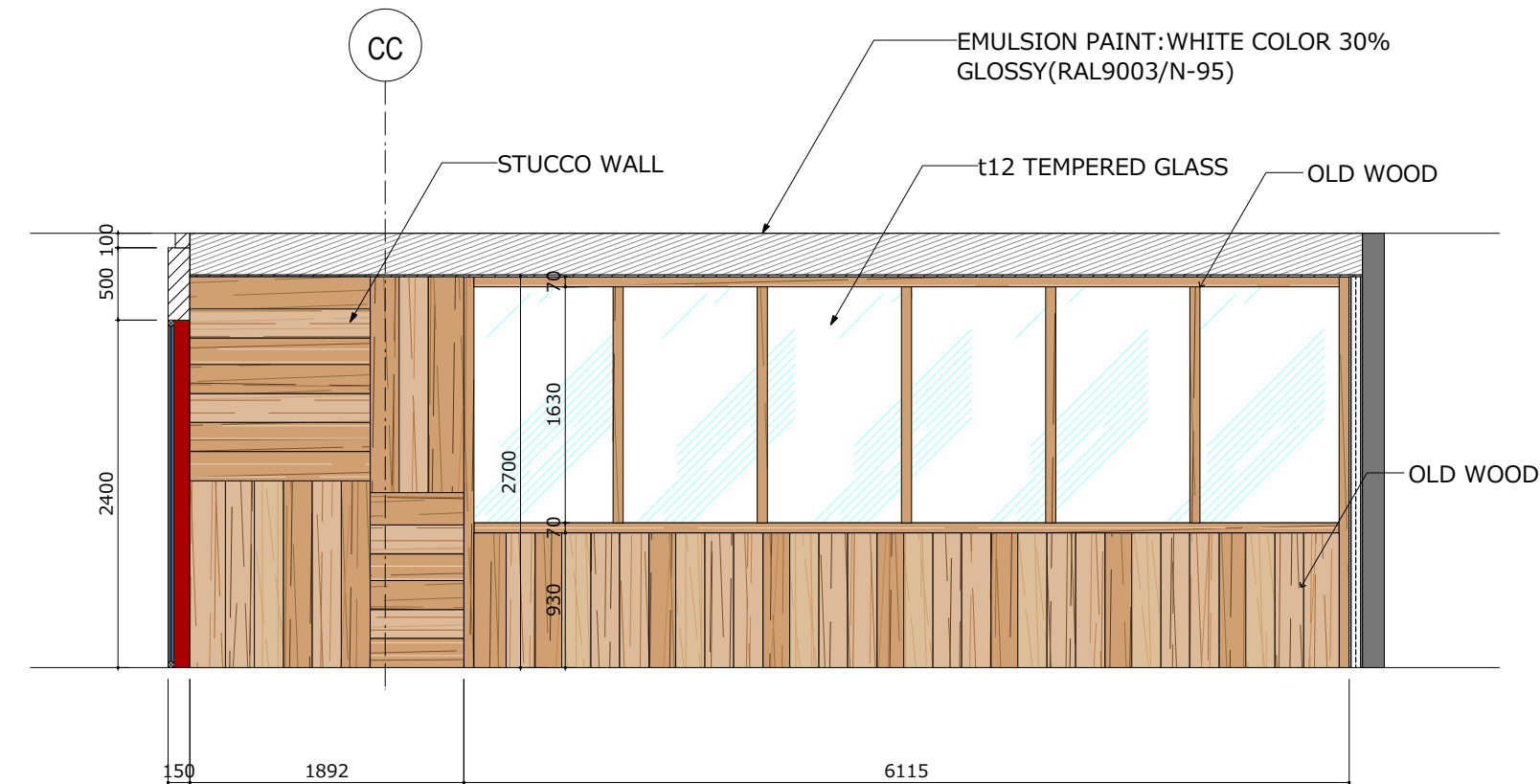
13 ELEVATION 1:50
