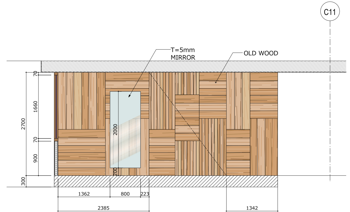
14 ELEVATION 1:50
