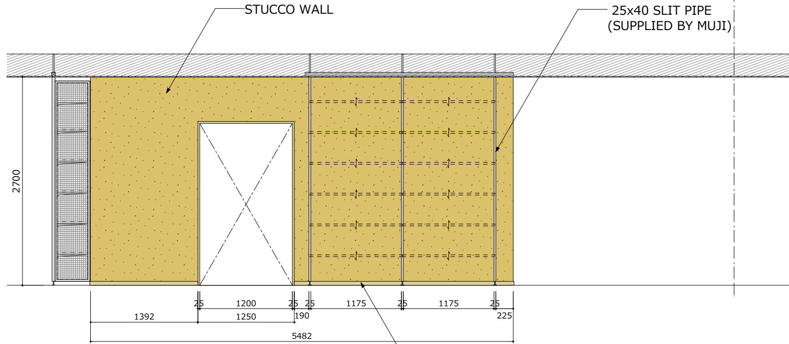
6 ELEVATION 1:50
