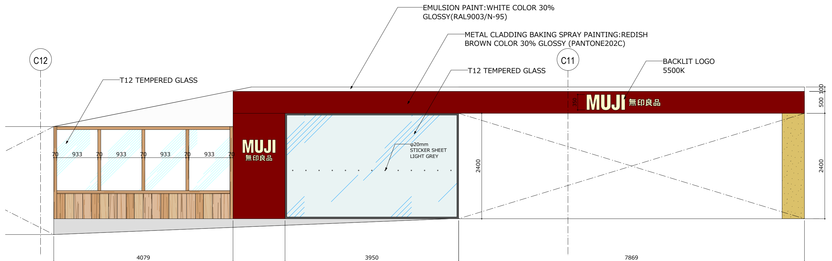
1 ELEVATION 1:50
