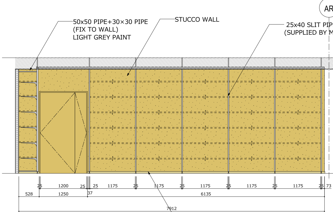
7 ELEVATION 1:50
