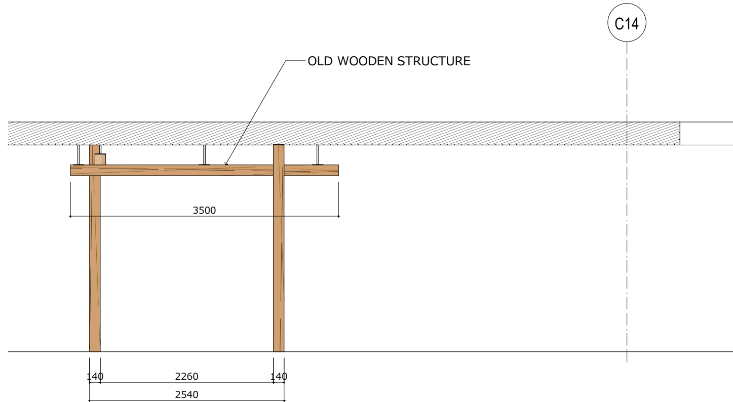
28 ELEVATION 1:50
