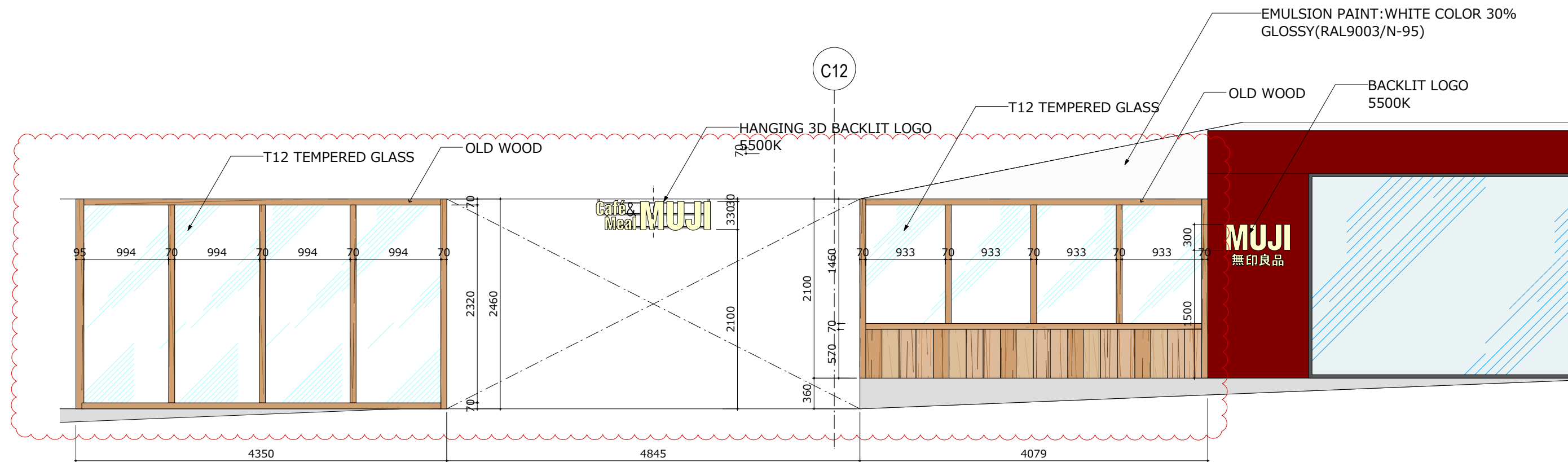
1 ELEVATION 1:50
