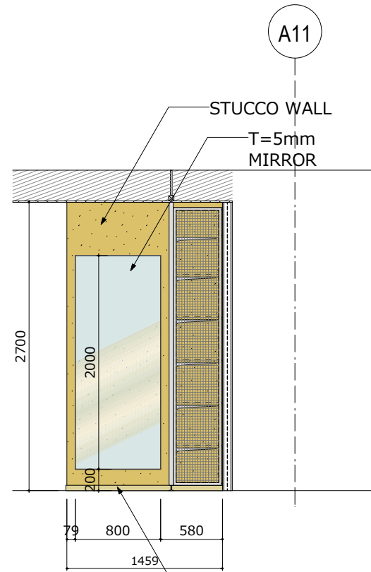
5 ELEVATION 1:50
