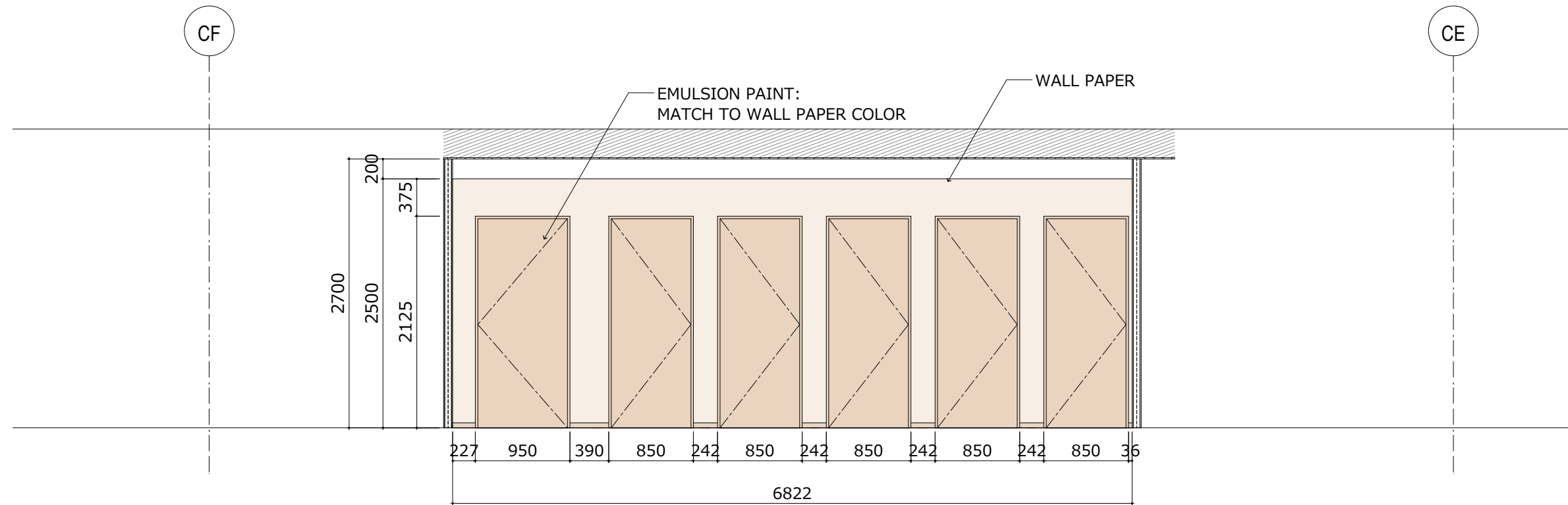
32 ELEVATION 1:50
