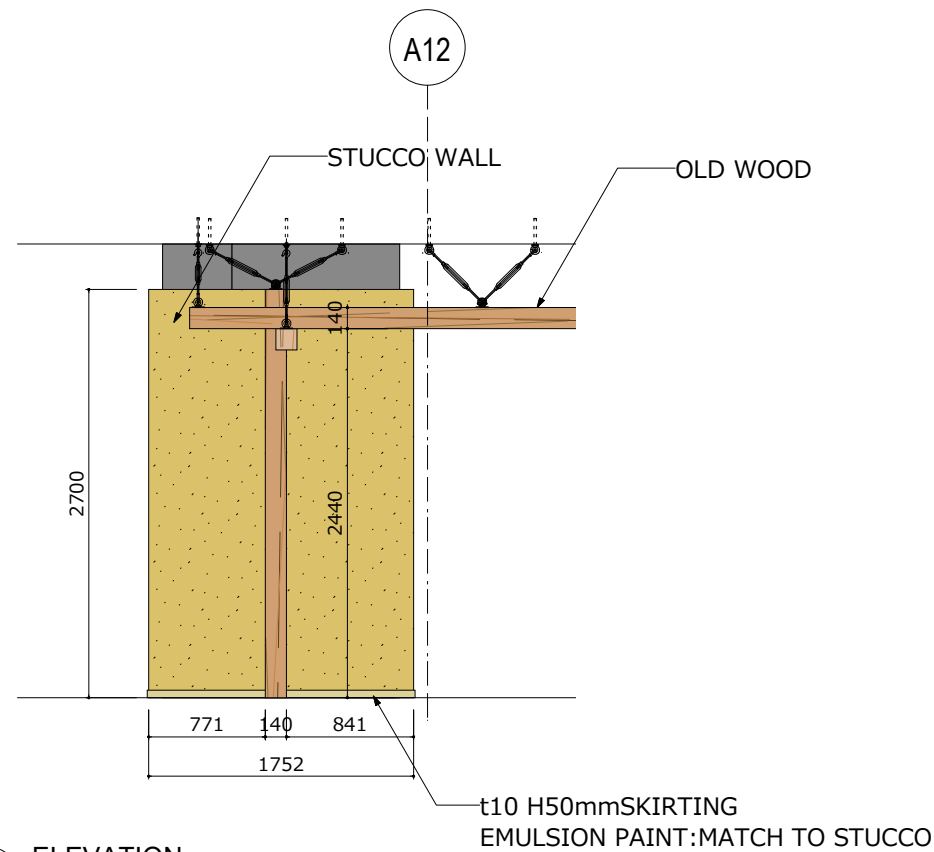
24 ELEVATION 1:50
