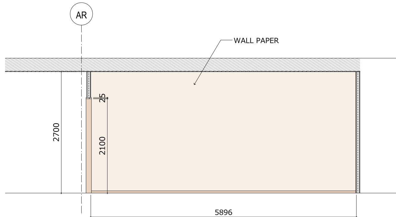
32 ELEVATION 1:50
