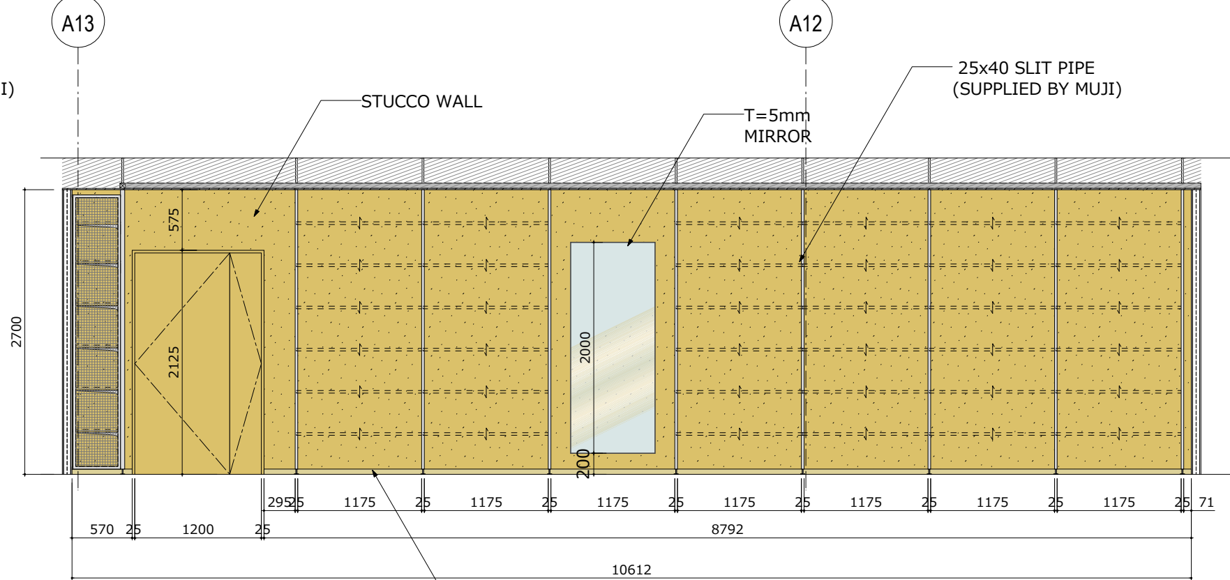
8 ELEVATION 1:50
