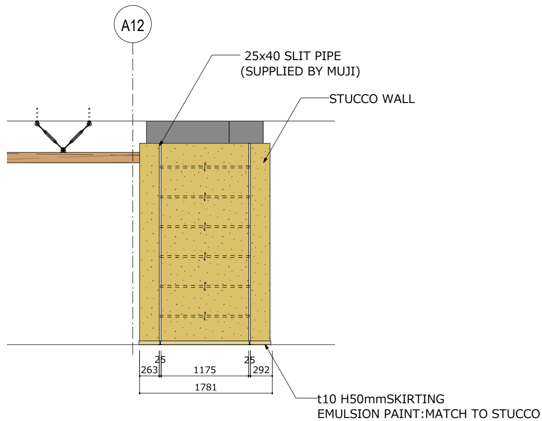
24 ELEVATION 1:50
