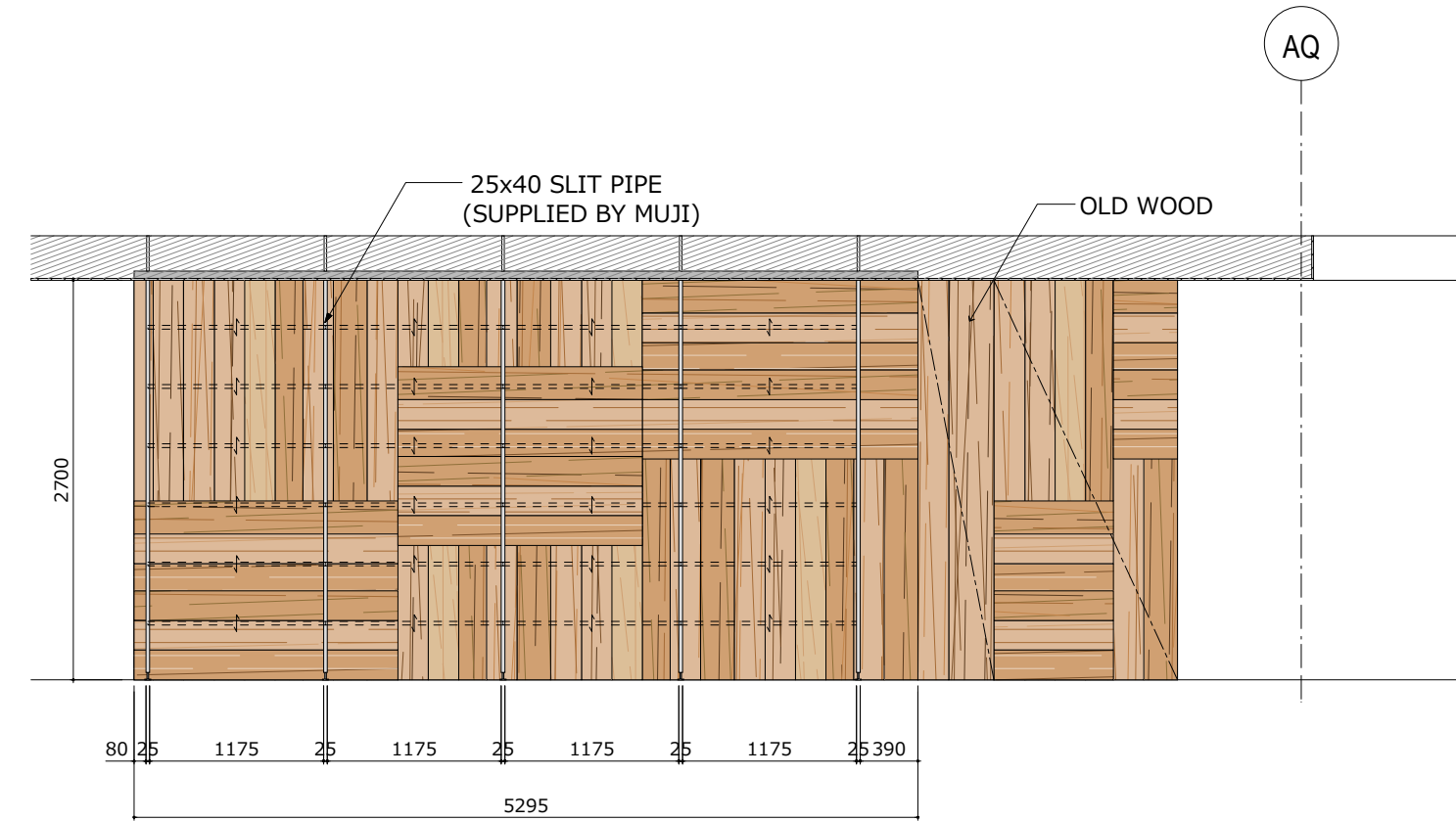
13 ELEVATION 1:50
