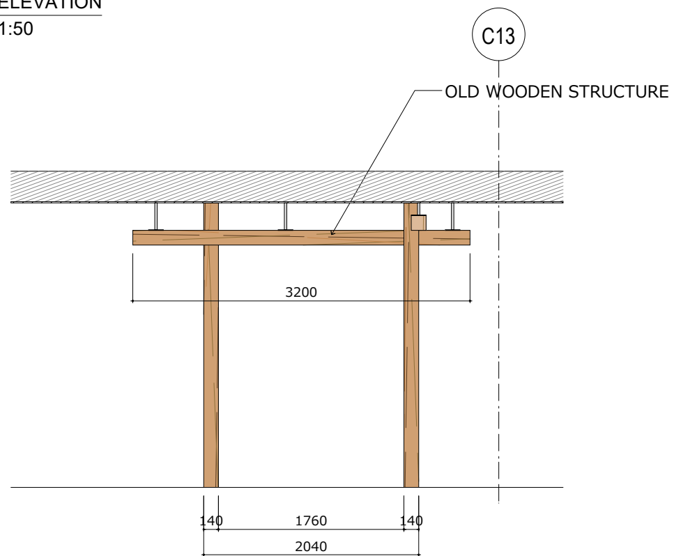
29 ELEVATION 1:50
